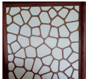
Voronoi | Voronoi
